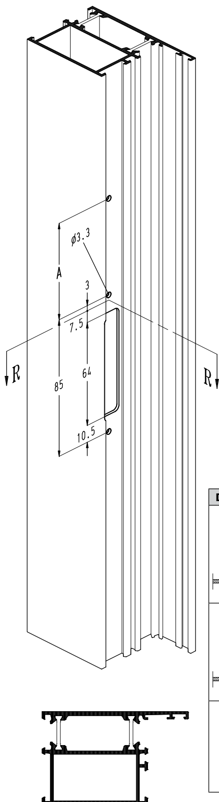
Kaderprofiel met kadergroef
