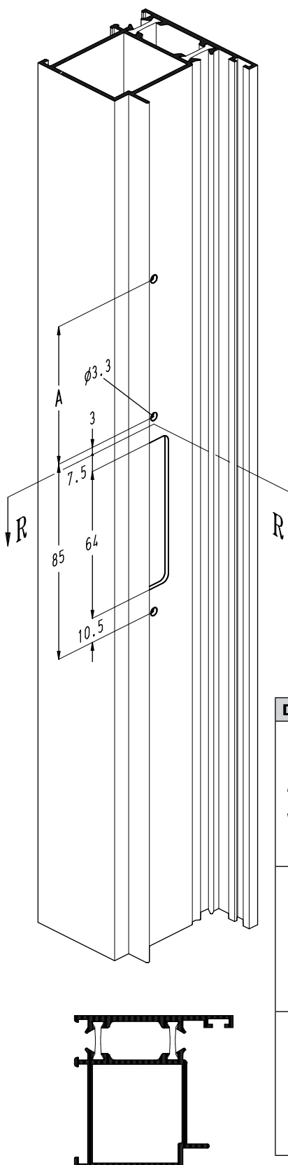
Kaderprofiel zonder kadergroef
