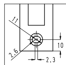
Bevestigingsgaten met een horizontaal regelbereik van 2,3 mm.
