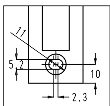
Bevestigingsgaten met een horizontaal regelbereik van 2,3 mm.
