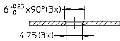
Doorsnede A-A schaal 2:1
