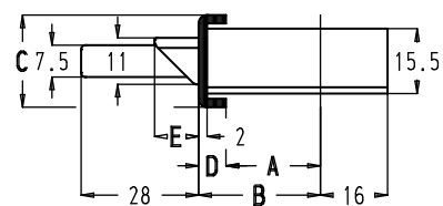
U-vormige voorplaat
