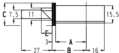
Vlakke voorplaat
