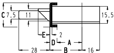
U-vormige voorplaat
