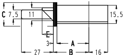
Vlakke voorplaat
