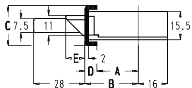
U-vormige voorplaat
